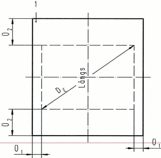
EN 1337-1, Nr. 1.1 Elastomerlager
